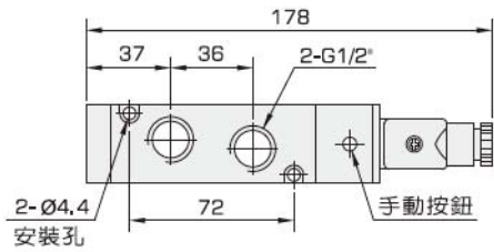
● VE4140 單線圈
