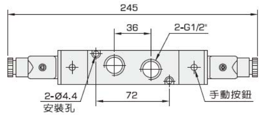
● VE4240 雙線圈
