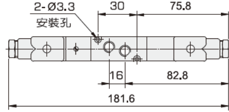
● VE1210 雙線圈
