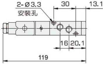
● VE1110 單線圈
