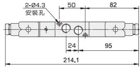
● VE3230 雙線圈
