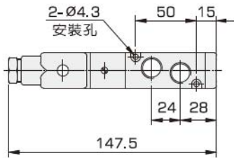
● VE3130 單線圈
